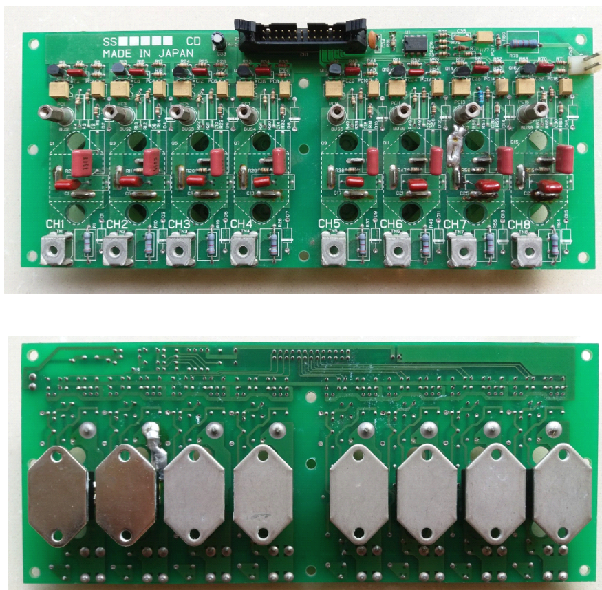
图 1 日本浅野真空成型机加热驱动板正、反面照片
